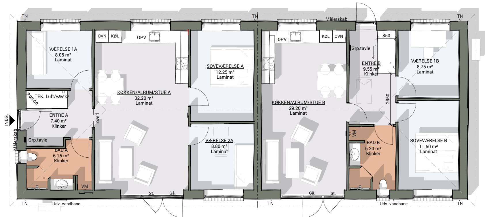
Plantegning 1 : 100
